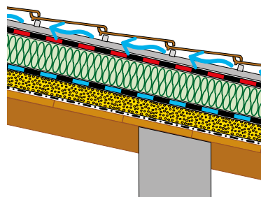
Tetto ventilato
