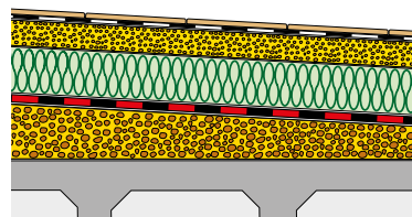
Tetto rovescio
