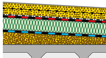
Tetto caldo
