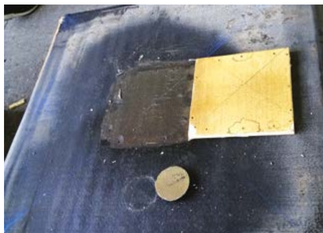
Campione di Lecamix dopo il test di pull-out secondo ANSI/SPR11A-1-2010.
