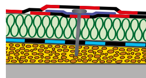
Esempio di fissaggio meccanico puntiforme sotto sormonta.
